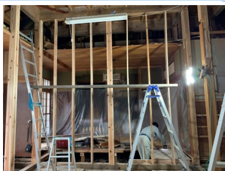
耐震およびリフォーム工事 天井、壁、床を解体、基礎を打ち 耐力壁を作っていきます。
