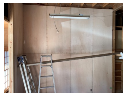
耐力壁完成☆土台から横架 材までの長さがある場合、構 造用合板補強が有効です。
